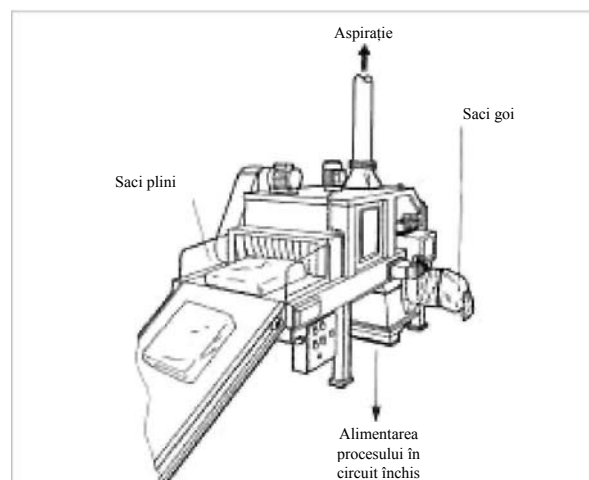
Figura I.5 – Mașină de vidare a sacilor*
