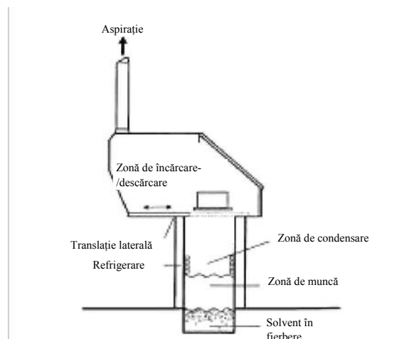
Figura I.7 – Cuvă de deairesare în fază de vapori*
