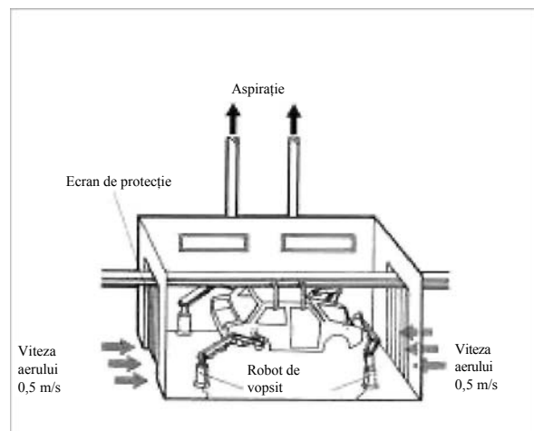
Figura I.3 - Tunel de vopsire*
