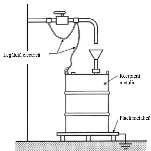
Figura I.23 – Legătură echipotențială și legare la pământ la transvazarea lichidelor inflamabile
