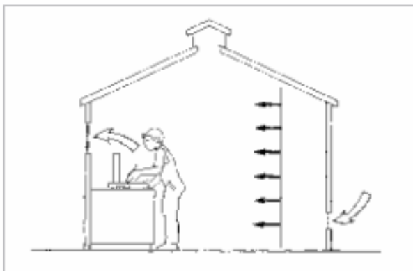
Figura I.18 – Situație corectă
